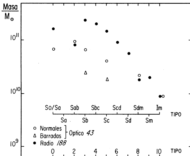
Fig. 2. Promedios de masas totales, ópticas y de radio con respecto al tipo morfológico desde S0/Sa hasta irregulares. Los valores obtenidos en radio son mayores que los ópticos en las espirales. En las irregulares son comparables las radio-masas y las masas ópticas. La tendencia de las espirales tempranas de tener menor masa de radio era ya aparente.
