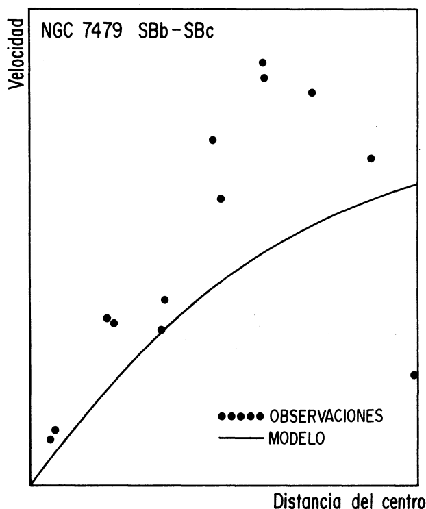
Fig. 4. Los puntos dados en NGC 7479, galaxia barrada típica SBb-SBc, dan una curva lineal desde -52'' hasta +55'' . No hay ajuste alguno con la expresión analítica de Brandt. La curva teórica no describe a las galaxias barradas.
