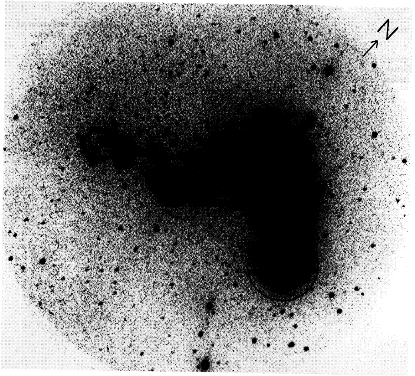
Fig. III: Fotografía en H\alpha de la Nube Menor de Magallanes; se indica una región de interés descrita en el texto.
