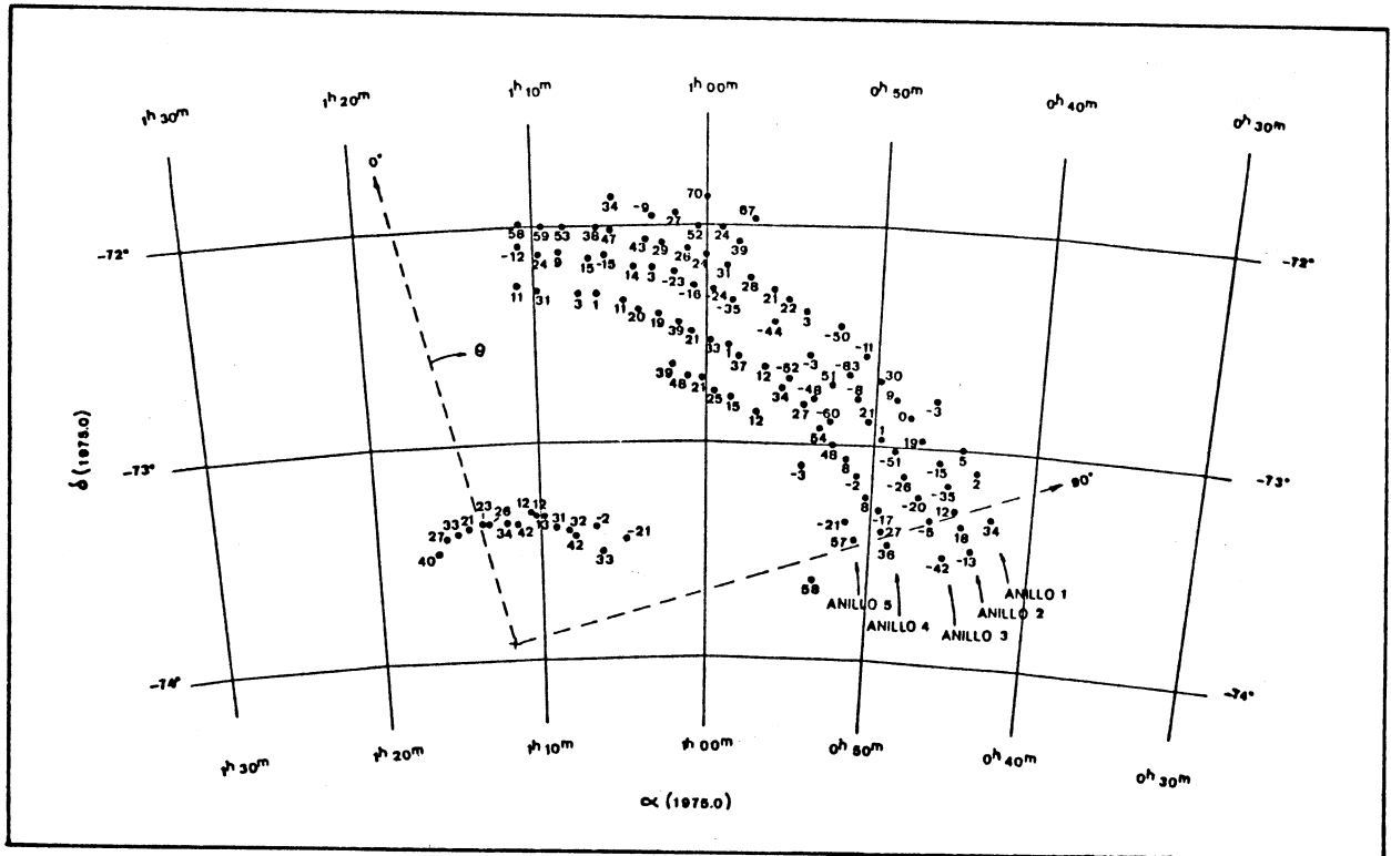
Fig. I: Velocidades radiales medidas, referidas al centro galáctico.
