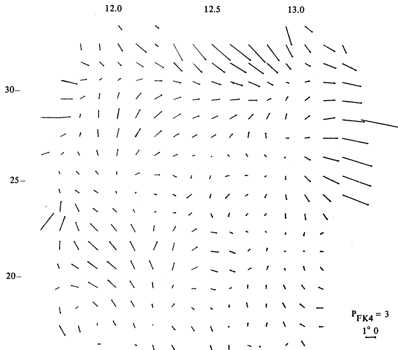
Fig. 1. Representación de los errores sistemáticos entre catálogos AGK3 y FK4 al promediar por zonas de 1^\circ \times 1^\circ las posiciones de las estrellas obtenidas en la reducción del área 1a.
