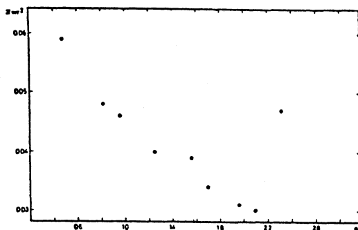
Figura 3. Parámetro de calidad de las soluciones fotométricas de FM Velorum.
