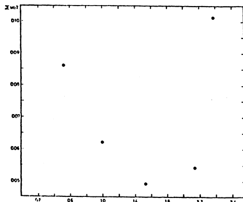
Figura 3. Parámetro de calidad de las soluciones fotométricas de FM Velorum.
