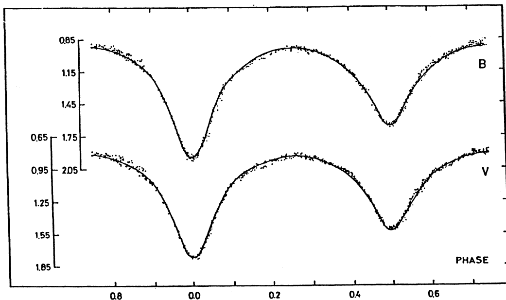
Figura 2. Curvas de luz teóricas y observadas de V676 Centauri.
