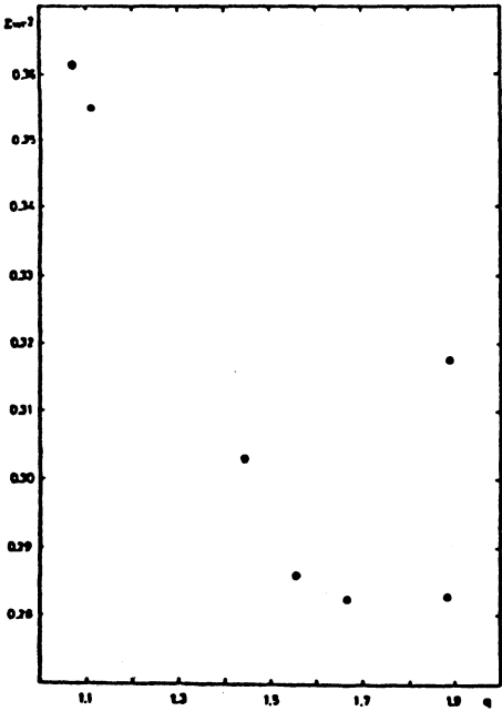
Figura 1. Parámetro de calidad de la solución fotométrica de V676 Centauri.
